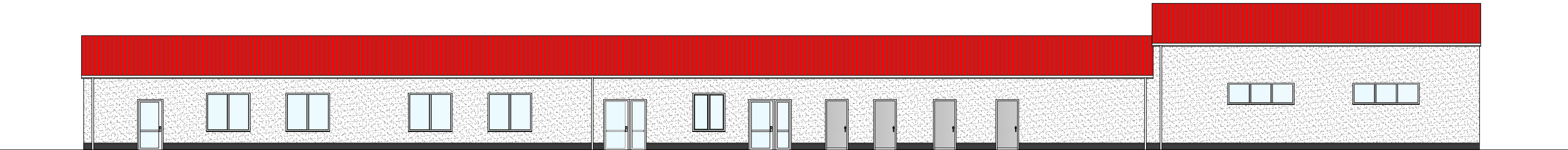
Ostansicht
