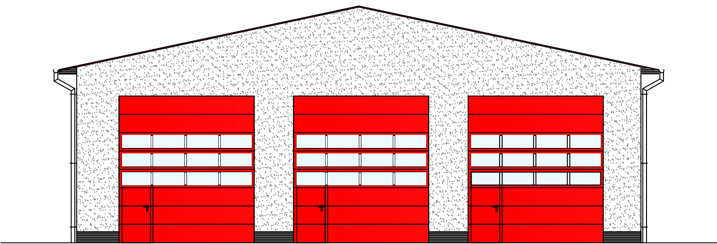
Nordansicht
