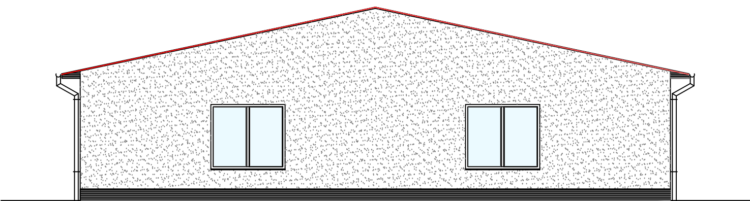
Südansicht
